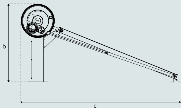
MẶT BÊN
